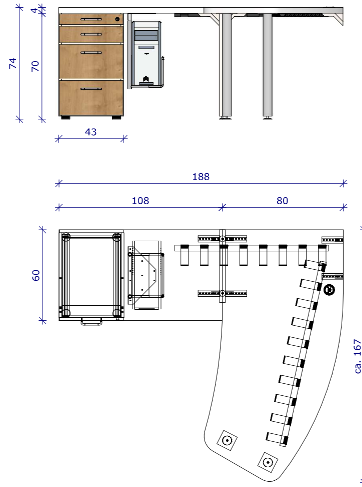
Pos. 2 Arbeitsplatzkombination
