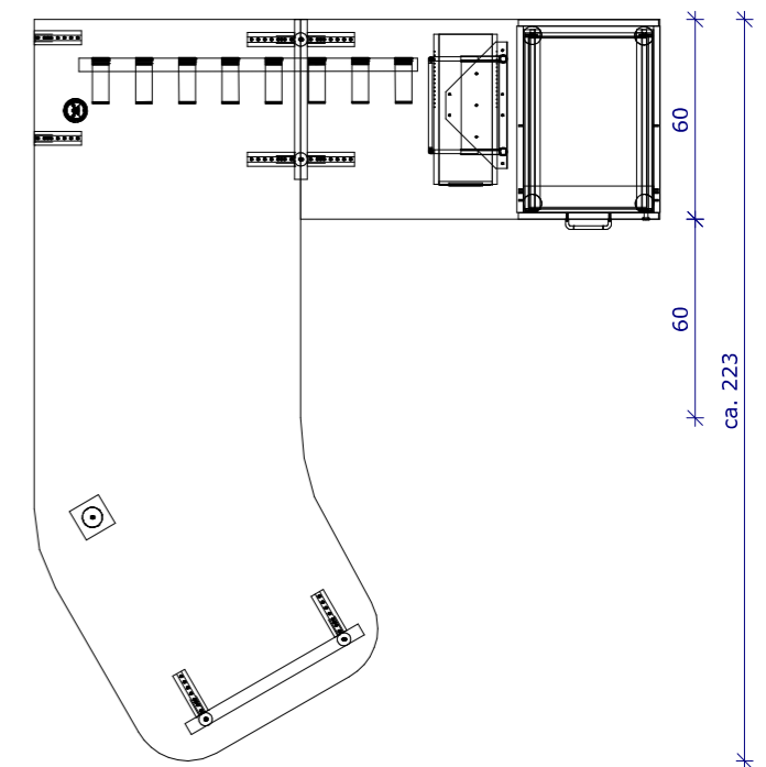
Pos. 6 Arbeitsplatzkombination
